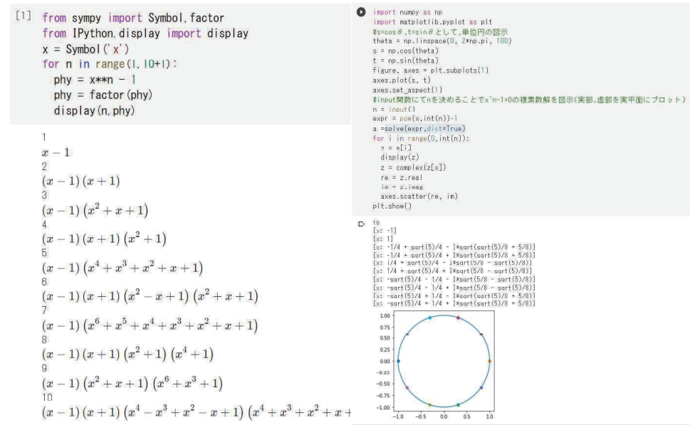
図 3: x^n - 1 の因数分解 図 4: 複素数解の図形的意味
