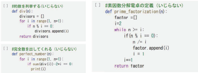
図 5: 利用するプログラム
