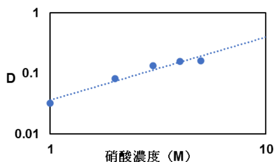
図1 TDdDGA を用いた Sb 分配比の硝酸濃度依存性
