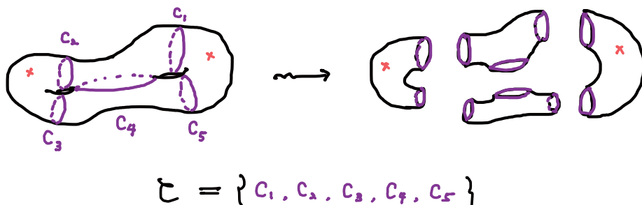
図 1. 点付き閉リーマン面 \mathcal{X}_{g,I} のパンツ分解 \mathcal{C}
