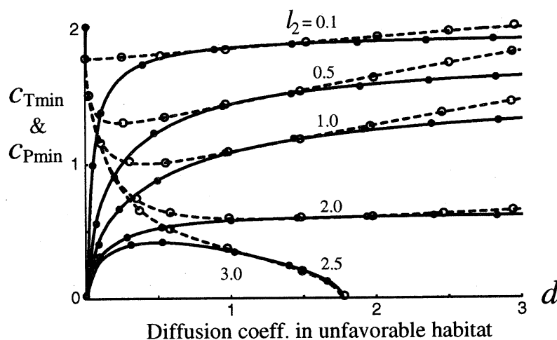
図2. a. 分断帯と平行に進む進行波の速度 c_{p\min} (点線) と分断帯を横断する進行波の速度 c_{T\min} (実線) の d , l_2 依存性. 黒丸と白丸は対応する数値計算の結果. \varepsilon = -0.5 , l_1 = 1 .
