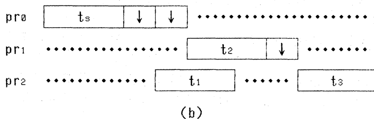
図2 FindMinPP の適用例
