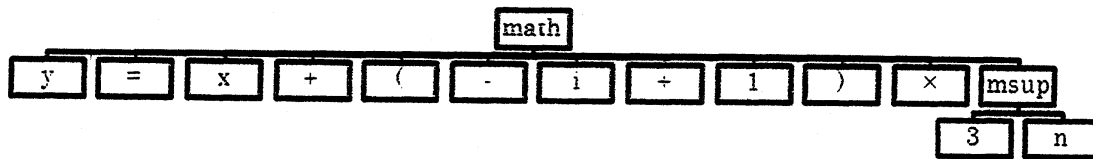
図 1: MathML の構造
