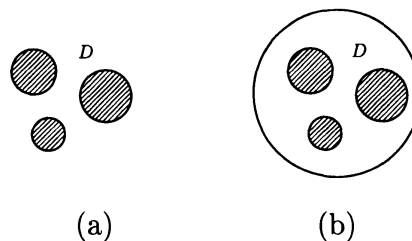
図 4: 正準円領域
