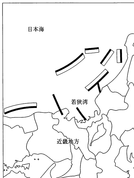
図5b：日本海近畿地方の沿岸と、沖で発生する津波を予測するために、「調査検討会」が検討した海底断層、および津波断層モデル（海底面に投影した矩形）。若狭湾内では2本だけ選定。検討会資料（2014より）。沖合の東北東―西南西などの方向の断層は、日本海の家盆と陸を限るもの。
