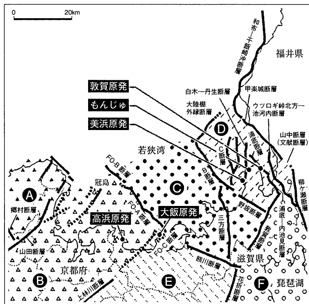
図5a：若狭湾とその周辺の地盤ブロック（A～F）と、それらの境の地断層。点線は想定されねばならないもの。原発の所在地を記入。より沖の断層については図5b参照。
