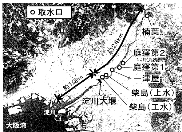
図1 淀川大堰および取水口位置
