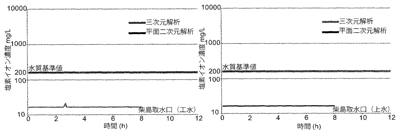
図16 取水影響評価河川流量 3000\text{m}^3/\text{s} (左：工水, 右：上水)
