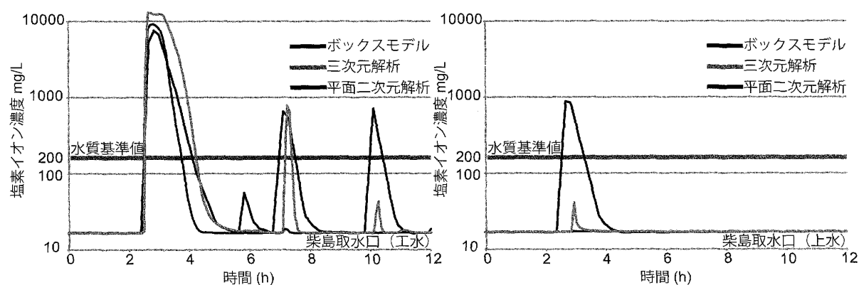
図14 取水影響評価河川流量 500\text{m}^3/\text{s} (左：工水, 右：上水)
