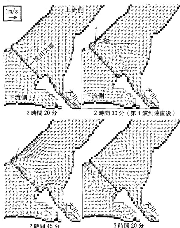
図6 淀川大堰近傍の流速変化(河川流量 196\text{ m}^3/\text{s} )
