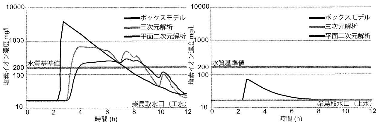
図12 取水影響評価河川流量 62\text{m}^3/\text{s} （左：工水，右：上水）
