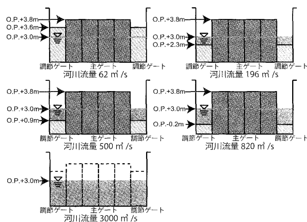
図3 淀川大堰天端高
