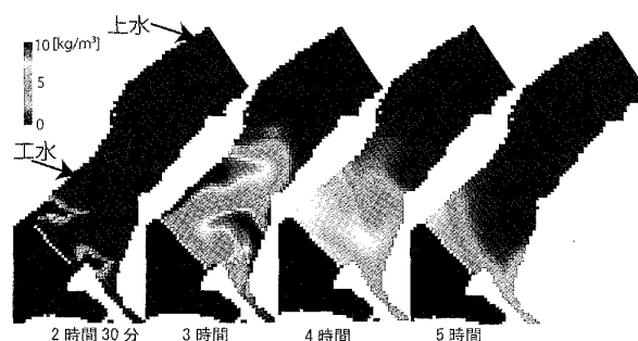
図 10 三次元塩水挙動解析結果河川流量 196\text{m}^3/\text{s}
