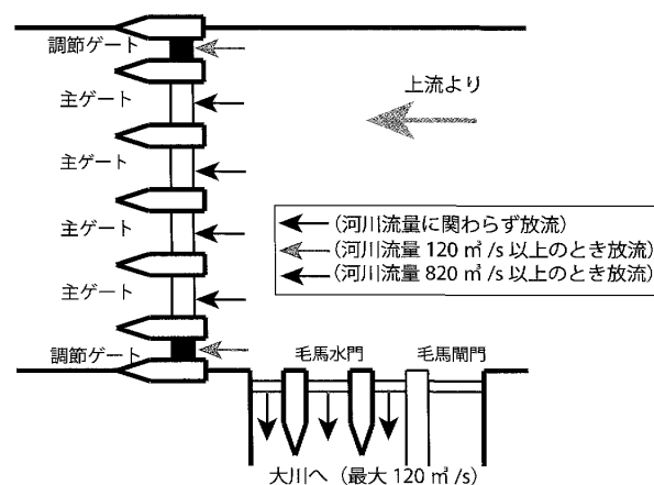
図2 淀川大堰模式図
