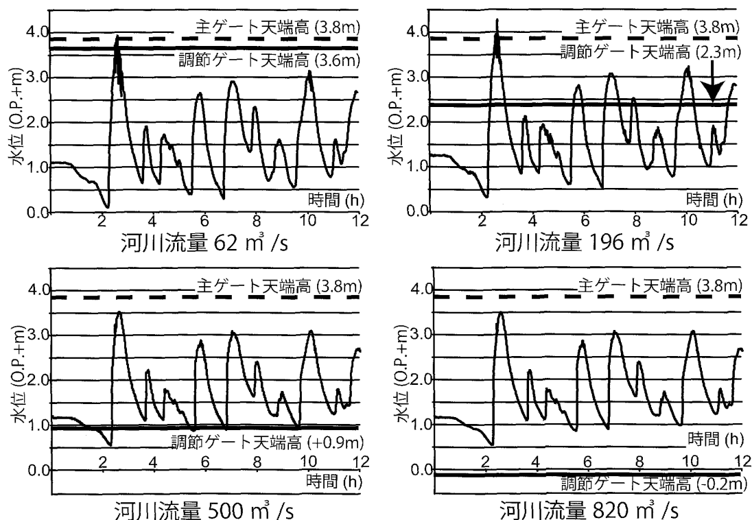
図5 淀川大堰下流位置での水位変化
