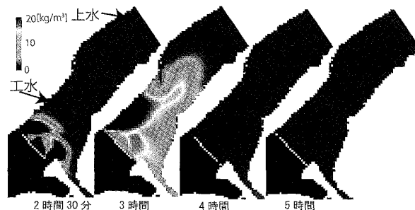
図 11 三次元塩水挙動解析結果河川流量 820\text{m}^3/\text{s}
