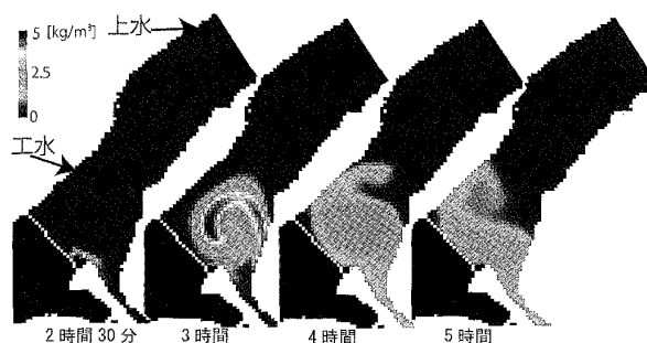
図 9 三次元塩水挙動解析結果河川流量 62\text{m}^3/\text{s}
