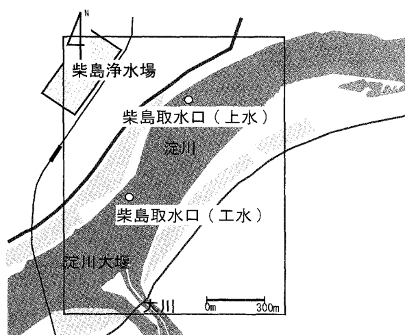
図 8 詳細解析の対象領域
