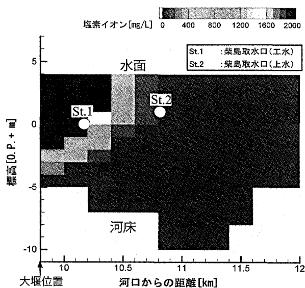
図7 鉛直二次元塩水挙動解析結果（河川流量 196 \text{ m}^3/\text{s} ）
