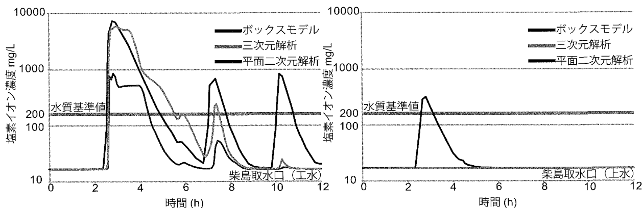
図13 取水影響評価河川流量 196\text{m}^3/\text{s} （左：工水，右：上水）
