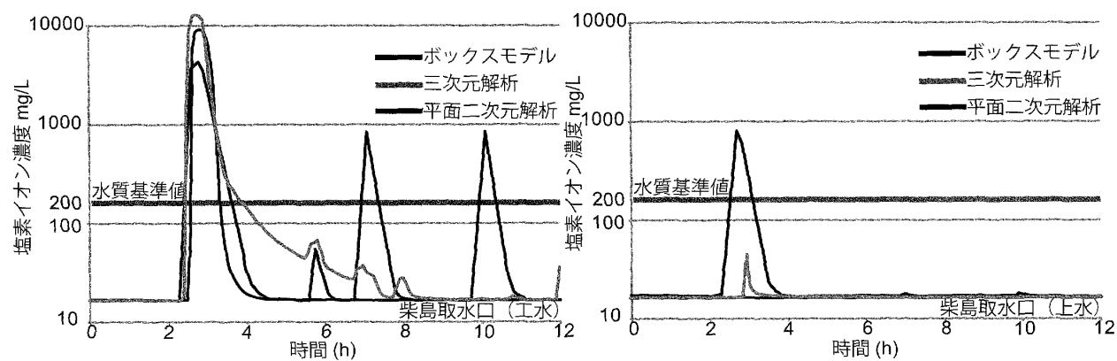
図15 取水影響評価河川流量 820\text{m}^3/\text{s} (左：工水, 右：上水)
