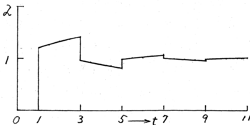
図 2 \mathcal{L}^{-1} (s \cosh \sqrt{s^2+1})^{-1}
