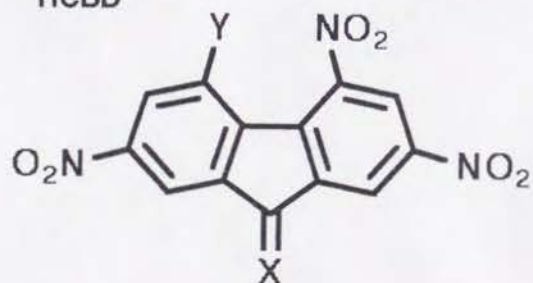
HCBT
