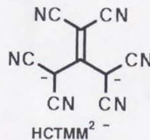
CF -
