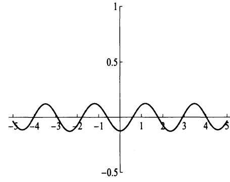
(d) \text{Im } \varphi_5^{ST}
