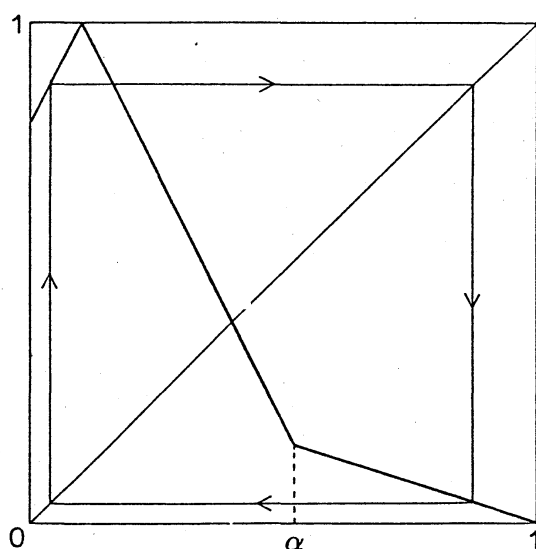
図11(a) 安定な2周期軌道
