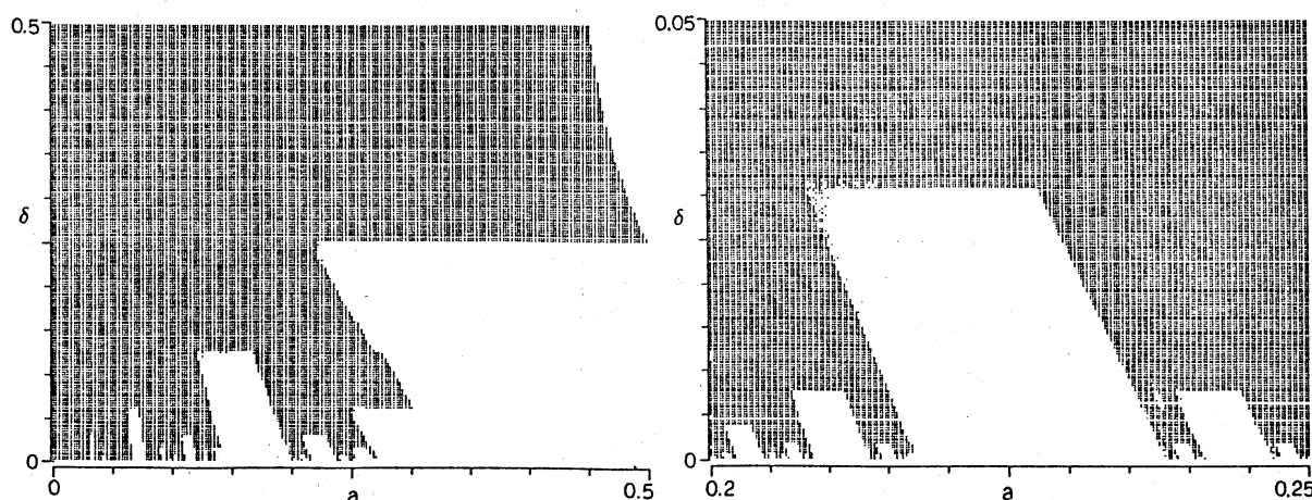
図10(a),(b) カオスの存在する領域
