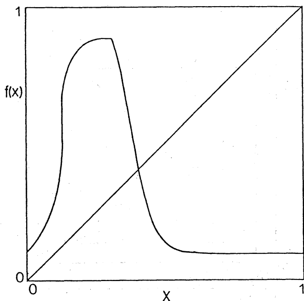
図1 B-Z写像
