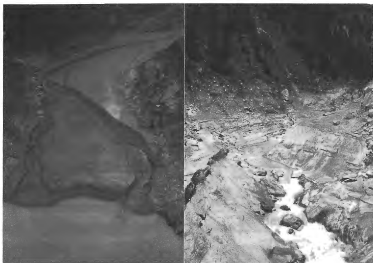
写真—3 ゲビデムダム（Gévières）の貯水池内に形成された水みち（フラッシング排砂水路）（EOS） （貯水池末端のデルタ堆積部（水位低下途中）、貯水池内（完全水位低下時））
