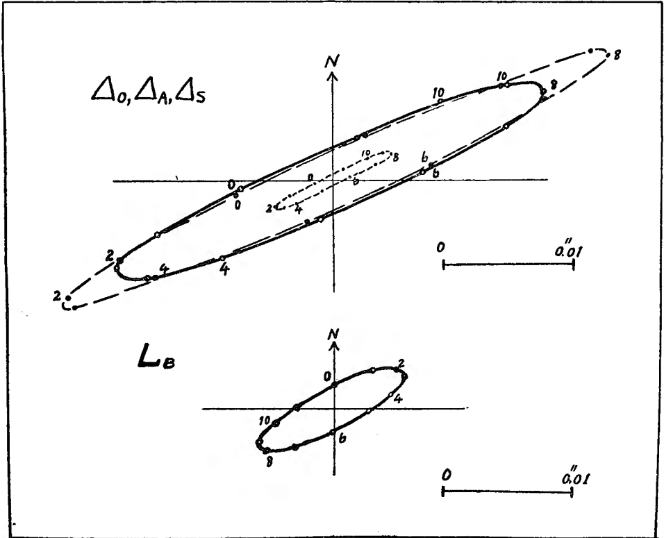
第 五 圖 (別府—阿蘇)潮汐圖 ( \Delta_A, \Delta_S, \Delta_{\text{別-阿}}, L_R )
