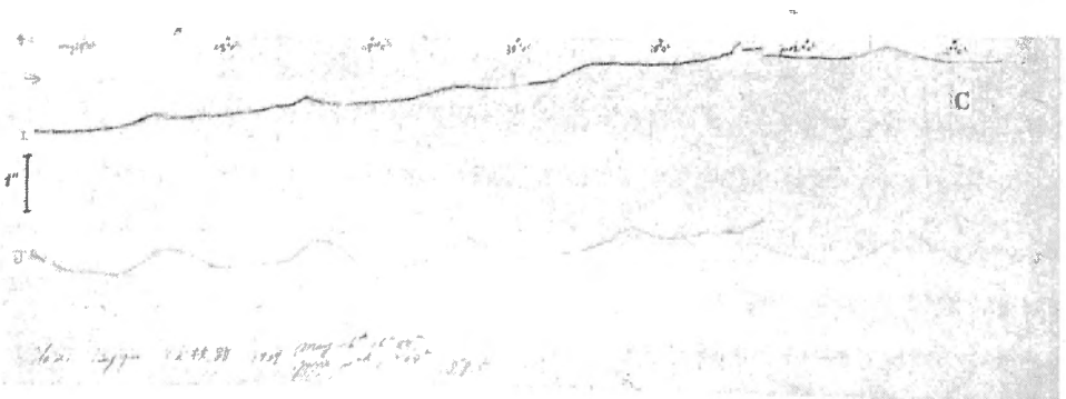
C. 高女跡 (昭和14年5月26日—6月2日)
