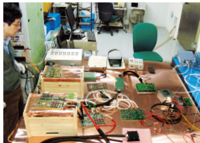
写真1: 机上で複雑にケーブル接続されている各観測ボード
