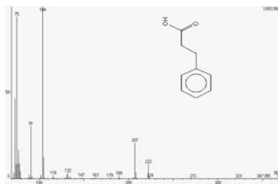
図 11 hydrocinnamic acid のマスペクトルと量的変化 入した時期を示す
