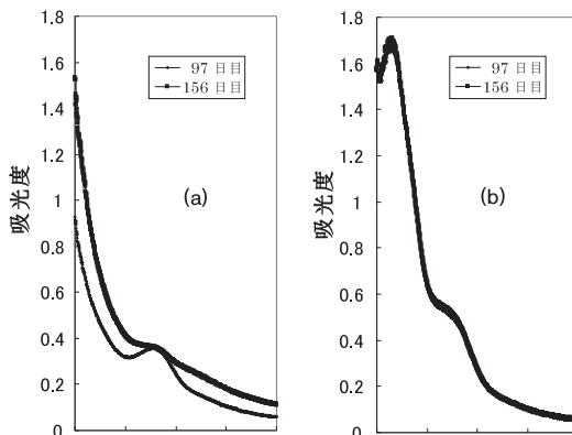
図7 酸可溶性リグニンの変化 (a) 硫酸塩還元条件 (b) molybdate 添加条件
