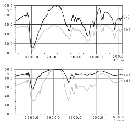
図9 硫酸塩還元条件におけるリグニンの赤外スペクトル変化 (a) クラースンリグニン 97日目 (b) クラースンリグニン 156日目 (c) APPL 97日目 (d) APPL 156日目
