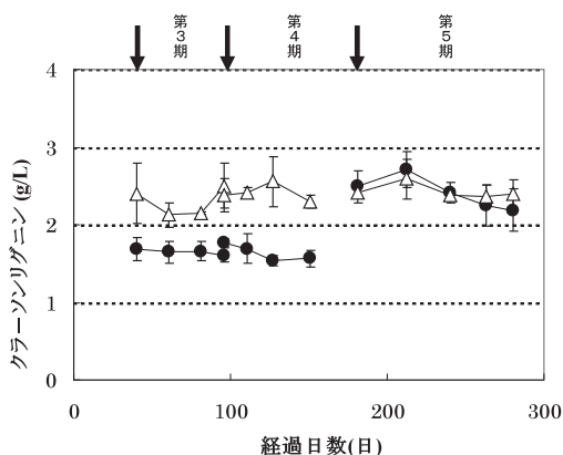
図6 クラークソンリグニンとして定量された高分子リグニン画分の濃度変化 (●：硫酸塩還元条件 △：molybdate 添加条件) 縦線は標準偏差を、矢印は硫酸塩と基質を再投入した時期を示す
