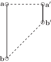
図 4: D_2^{(2)} D_1^{(1)}(\mathbf{a}) ( a'_1 \geq a_1 かつ a_2 > a''_2 のとき)
