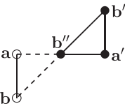
図 3: D_2^{(2)} D_1^{(1)}(\mathbf{a}) ( a'_1 \geq a_1 かつ a''_2 \geq a_2 > a'_2 のとき)
