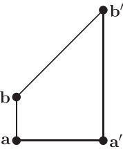
図 2: D_2^{(2)} D_1^{(1)}(\mathbf{a}) ( a'_1 \geq a_1 かつ a'_2 \geq a_2 のとき)
