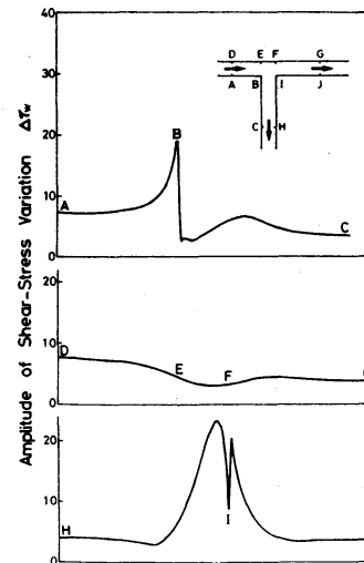
図 17 剪断応力の変動幅 ( R=64, T=10, \psi_s=0.5 )
