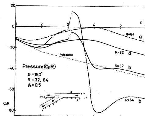
圖 8 壓力分布 ( \theta=150^\circ, \psi_s=0.5 )
