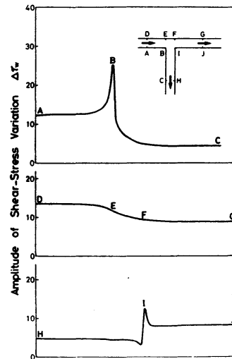
図 14 剪断応力の変動幅 ( R=32, T=1, \psi_s=0.35 )
