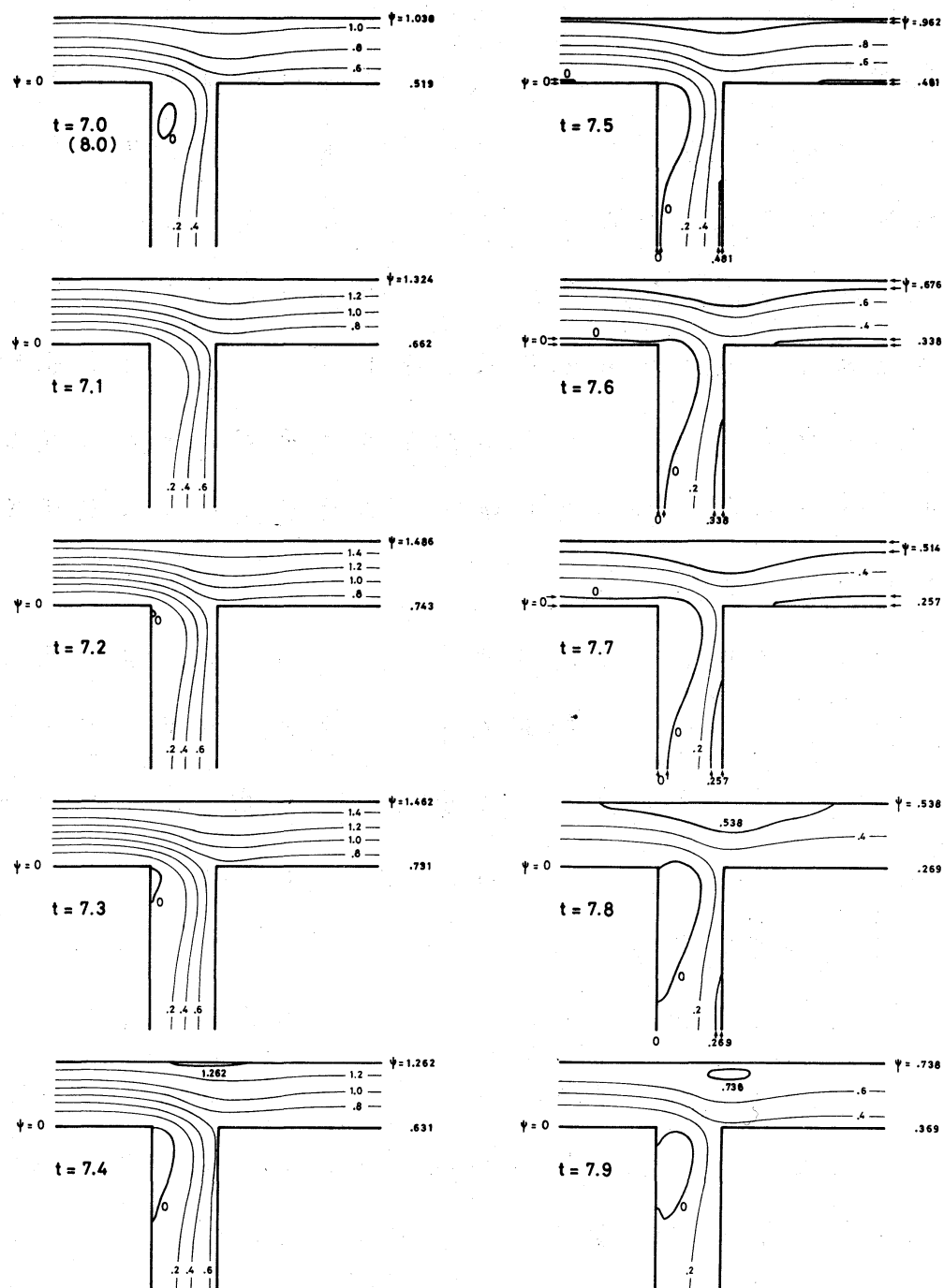
圖 10 流線 ( R=64 , T=1 , \psi_s = 0.5 )
