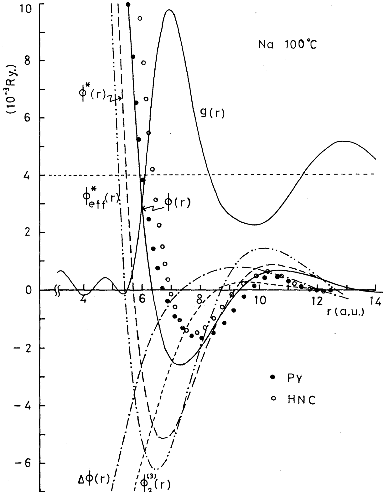
図3. Na のイオン間相互作用。 \phi(r) , 2次摂動計算: \phi^*(r) + \phi_2^{(3)}(r) : \phi_{\text{eff}}^*(r) = \phi^*(r) + \Delta\phi(r) : PYおよび HNC, S(q) の実験データ 27 から Percus-Yevickおよび Hypernetted chain 方程式にもとづいて計算されたポテンシャル, なお \Delta\phi(r) には図11の(1)の結果を用いた。
