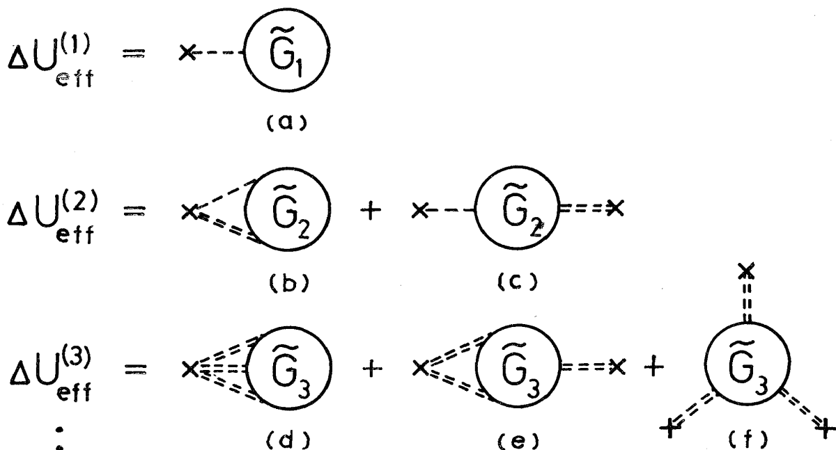
図 1. \Delta U_{\text{eff}}^{(n)} のダイヤグラム表示, 点線, W_0(q) : 2 重の点線, W(q) = W_0(q) / E(q) : \times 印, \rho_i(\mathbf{q}) = \sum_j \exp[-i\mathbf{q}\mathbf{r}_j] : \tilde{G}_n , 電子ガスの既約な n 体グリーン関数。ここでは \rho_i(\mathbf{q}) を m 個含むダイヤグラムは m 体のイオン間相互作用だけで表わされるように, イオンの座標についての和に制限をつけてある。(本文参照)。また波状についての和および各ダイヤグラムの数因子は省略してある。
