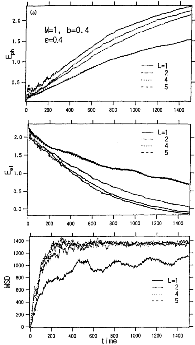
図 2: ランダム系に多色の外摂動が加わった場合 M=1, L \geq 2, \epsilon=0.4 。
