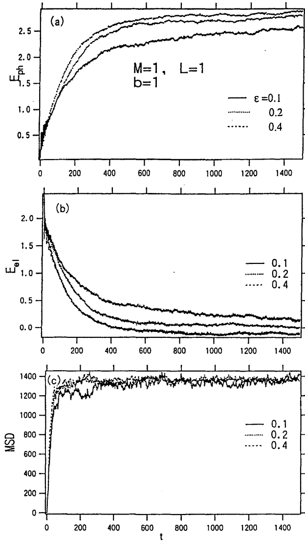
図 1: ランダム系に単色の外摂動が加わった場合 M=1, L=1 。
