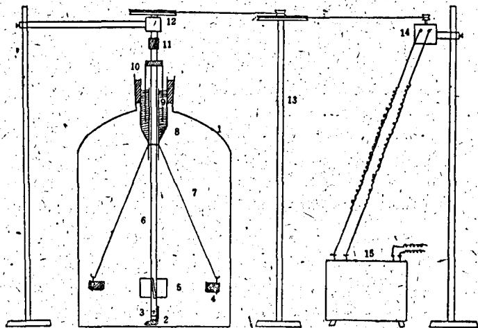
第1図 燻蒸装置
