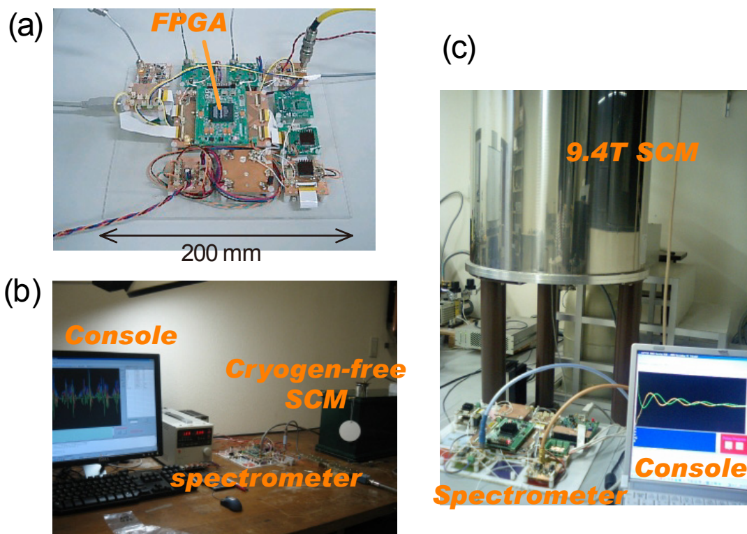
図3. (a) OPENCORE NMR Spectrometer の外観. (b) 磁場可変無冷媒超伝導電磁石(Cryogen-free SCM)を用いた使用例. (c) 9.4 T 超伝導電磁石(SCM)を用いたNMR システム. 制御指令およびNMR 信号データの転送にはUSB を用いている. コンピュータディスプレイには, 独自に開発した OPENCORE NMR 測定ソフトウェアのコンソール画面が映っている.
