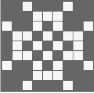
図 24: 変形したチェスボード
