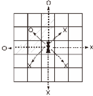
図 13: 龍王の動き
