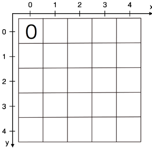
図 3: (0,0) の Grundy 数
