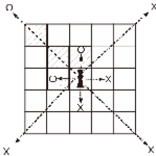
図 11: 龍馬の動き
