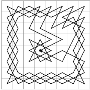
図 22: ナイトの動きをトレースしたもの ([18])
