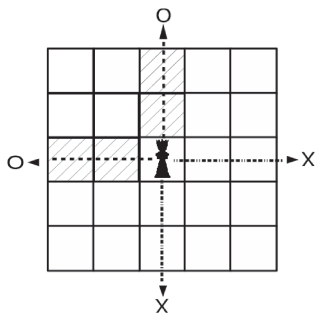
図 9: 飛車の動き
