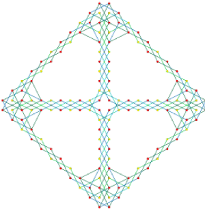
図 26: 2つのナイトによるナイトグラフ 図 27: 2つのナイトによるナイトグラフ
