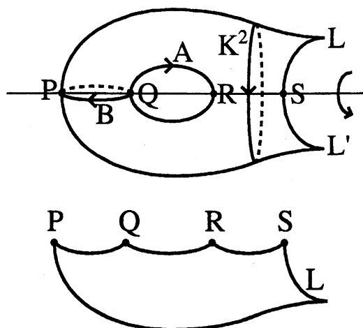
図 6: 2 点穴あきトーラスと (2, 2, 2, 2, \infty) -オービフォールド
