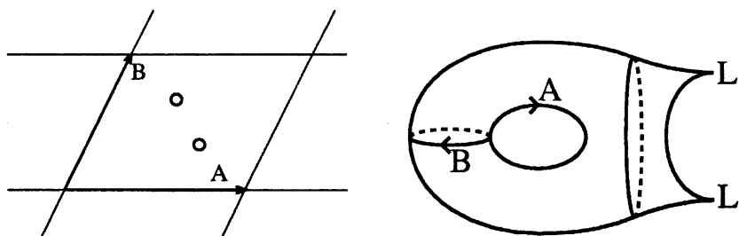
図 5: フックス型2点穴あきトーラス群
