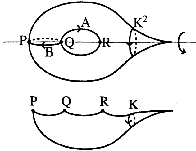
図 3: 1 点穴あきトーラスと (2, 2, 2, \infty) -オービフォールド.
