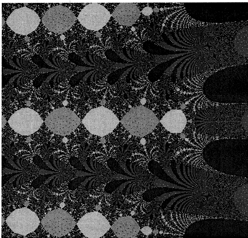
図 1: f(z) = \lambda ze^z のファトウ集合
