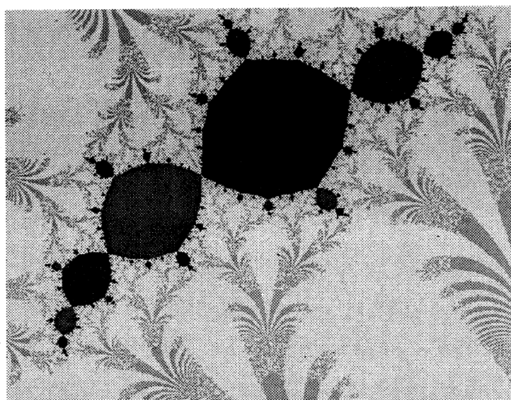
図 2: \lambda = 0.0577688 - 0.0721882i a = 4 - 2.8i
