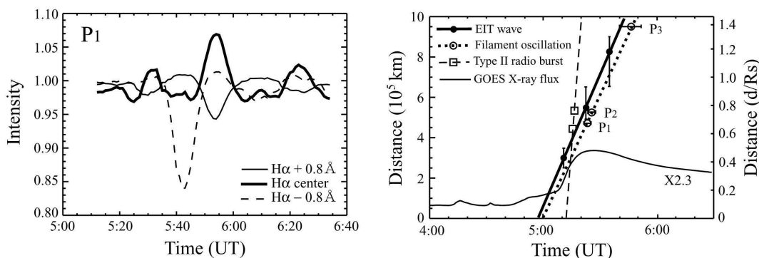
図: (左)H \alpha フィラメントの3波長(H \alpha , H \alpha + 0.8 Å: red wing, H \alpha - 0.8 Å: blue wing)による光度曲線。EIT waveがこのフィラメント上を通過したのは5:20 UT。その後、blue wing と red wing が交互に振動しているのがわかる。(右)EIT wave の波面位置と3つのフィラメント振動の位置及び開始時刻の関係。Type-II 電波バースト・GOES のX線強度の変化もプロットしてある。
