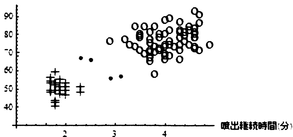
図 6.3 IC_\beta の推奨モデル (クラス数 k = 2 , 黒の 4 点が異常値と検出された)
