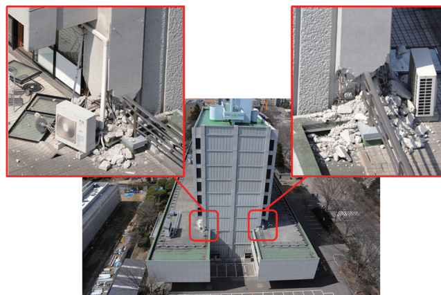
写真4 東北大学人間環境系研究棟の被害
