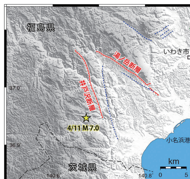
図2 4月11日M7.0いわき市南西部地震の地震断層の分布。井戸沢断層で最大2.3m、湯ノ岳断層で0.8mの上下変位(ズレ)を現地で確認。青破線は、既存の活断層(新編「日本の活断層」より)。
