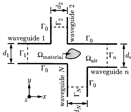
図 1 導波管 H 面回路結合部
