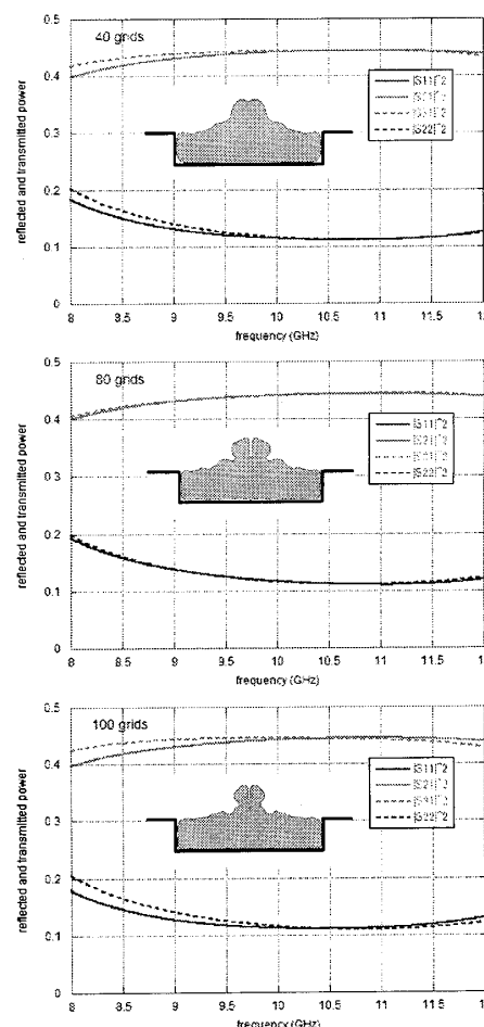
図3 最適化構造に対する入出力特性
