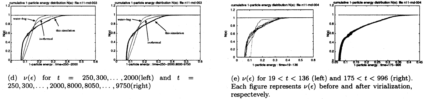
図 10: 1 粒子エネルギー分布 \nu(\epsilon) の時間発展
