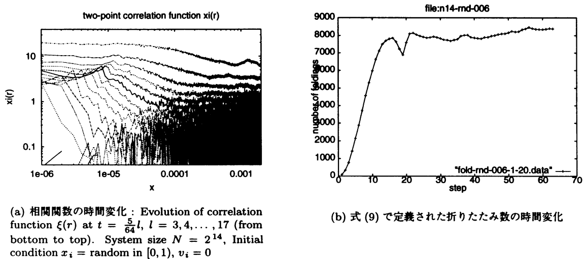
図 7: 2 点相関関数と 折りたたみ数の 時間変化
