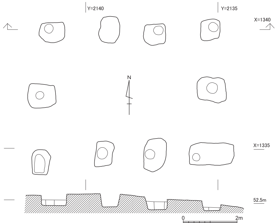
図63 建物S B 1 縮尺1/80
