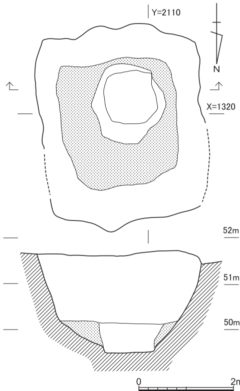
図62 井戸 S E 30 縮尺1/80
