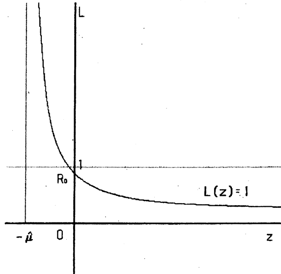
図 1: L の概形
