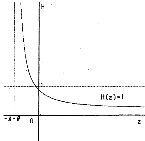
図 2: H の概形
