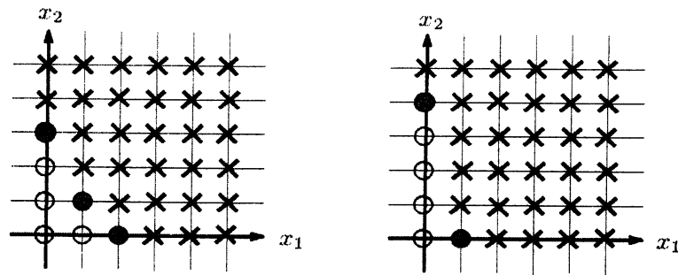
図 1: G_1 と G_2 の頭項による割り切れる項と割ることのできない単項の識別図
