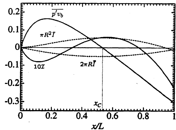
図3：境界層が主流部にするパワー \overline{p'v_b} と音響エネルギー流束の分布。ここで、 \pi R^2 \bar{I} , 2\pi R \tilde{I} はそれぞれ、主流部を流れる流束と境界層内を流れる欠損流束であり、 10I は全断面を流れる流束を10倍拡大して表示したものである。
