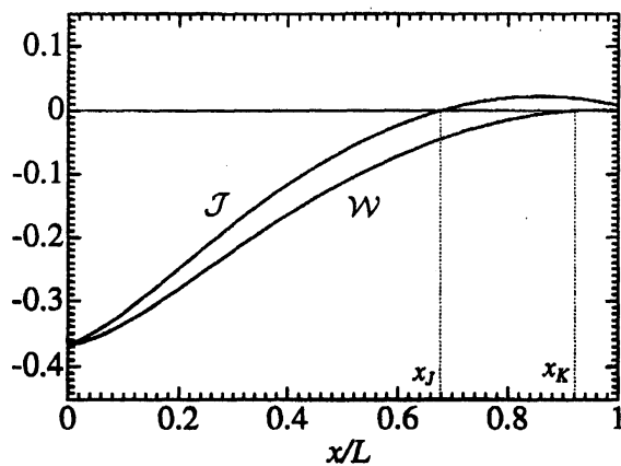
図4：管の全断面にわたる移流による熱流束 J とエンタルピー流束 W の分布。それぞれの正負が変わる位置を、 x_J, x_K で示す。
