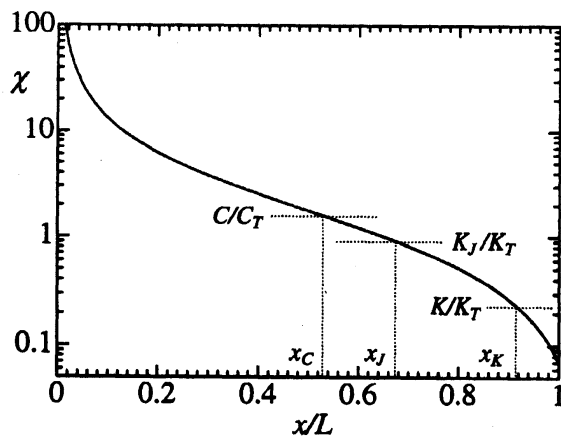
図2：管に沿った各位置での \chi の値。ここで、 \chi の値がそれぞれ、 C/C_T , K_J/K_T , K/K_T の値に等しくなる位置を、 x_C , x_J , x_K で示す。
