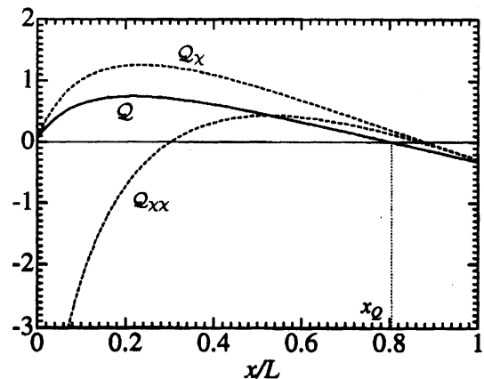
図5：管の側壁からの熱流束の分布。ここで、 Q と Q_{xx} はそれぞれ、(3.32), (3.25) で求めた量であり、 Q_x は (3.26) で \chi^2 を無視して求めたものである。
