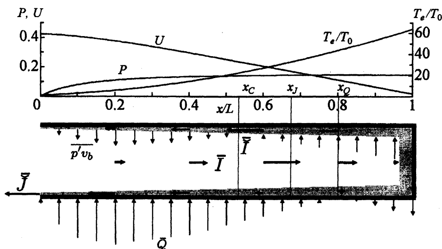
図6：主流部および境界層（グレー）を流れる音響エネルギー流束と熱流束の時間平均量の分布。矢印はその向きを、長さは概ね大きさを表す。両端の最大温度比を64とし、 P 、 U は圧力と流速の複素振幅を表すが、両者の位相は \pi/2 異なる。
