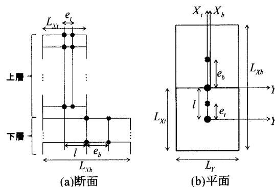
図1 セットバック建物
