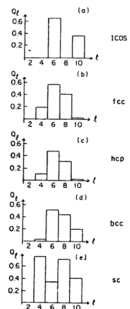
図3 いくつかの配置に対する Q_l 一番上が正20面体約12方向
