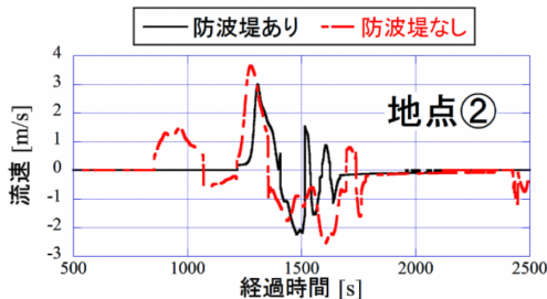
図-16 湾口防波堤の効果の検討（流速時系列1）
