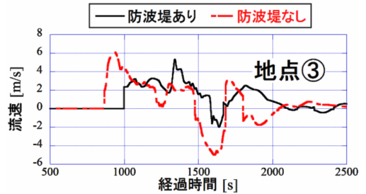
図-17 湾口防波堤の効果の検討（流速時系列2）
