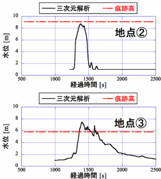
図-9 津波水位の時間変化例 (三次元解析)
