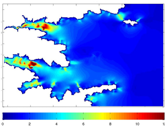
図-13 湾口防波堤なしの最大流速分布 (準三次元, 単位 m/s)
