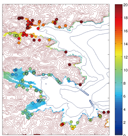
図-4 津波痕跡調査結果と解析結果の比較 (準三次元) (○: 痕跡調査結果, 濃淡: 解析結果, 単位: m)
