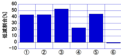
図-14 湾口防波堤による津波高さの低減割合
