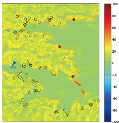
図-5 津波痕跡調査結果と解析結果の相対誤差 (準三次元) (○: 相対誤差, 濃淡: 地形勾配, 単位: %)
