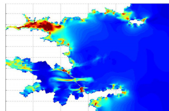
(a) 三次元解析結果
