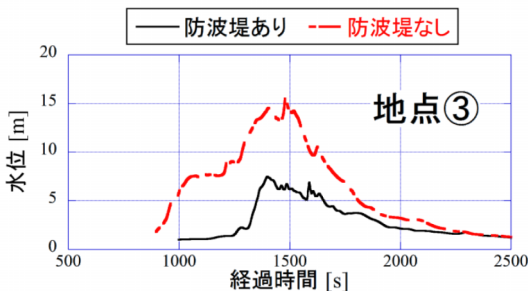
図-15 湾口防波堤の効果の検討（津波水位時系列）
