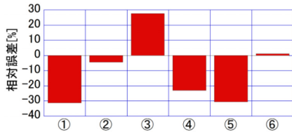
図-7 津波痕跡調査結果と解析結果の相対誤差 (三次元)
