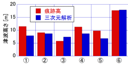
図-6 津波痕跡調査結果と解析結果の比較 (三次元)
