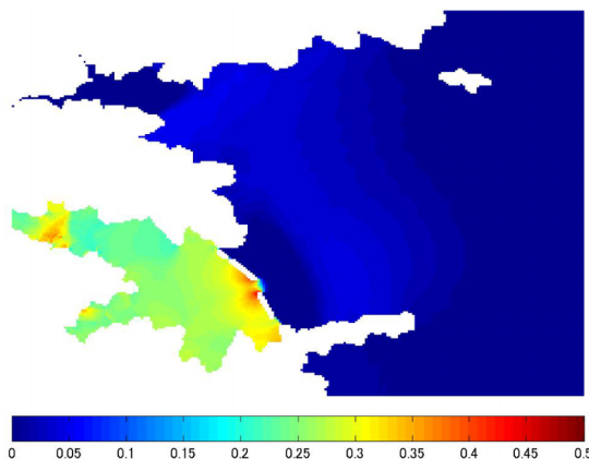
図-12 湾口防波堤による陸上部津波水位の低減割合
