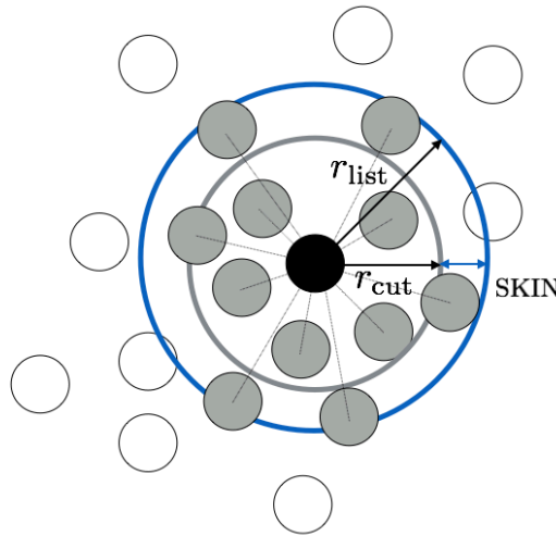
図 2.1 ベルレの近接リスト法 (VNL) の概念図: \text{SKIN} = r_{\text{list}} - r_{\text{cut}} , r_{\text{cut}} はカットオフ半径, r_{\text{list}} はリスト半径を表す. 灰色粒子は黒色粒子の近接リストに記憶されている粒子であり, 毎ステップリストを用いて相互作用を計算することが出来る. 白色粒子はリストの外にでており, 計算の必要の無い粒子である.
