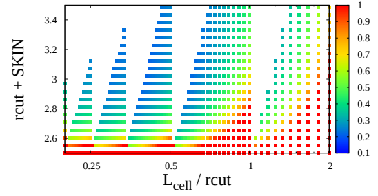
図 4.3 式 (4.3) の結果：計算時間の SKIN，セルサイズ依存性. T = 1.0 , \rho = 0.8 , r_{\text{cut}} = 2.5 としてそれぞれ粒子数を変化させている.
