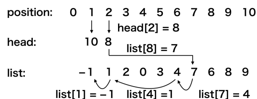
図 3.4 \text{head} 配列， \text{list} 配列のリンク構造の概念 図： \text{position}_2 のセルには \text{head}[2] = 8 ，つまり 8 番の粒子が先頭に入っている．さらに \text{list}[8] = 7 ，つまり 8 番粒子の次は 7 番粒子が入っている． \text{list} 配列が -1 を返すまでこれを繰り返す．
