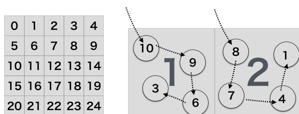
図 3.3 左：セルインデックス \text{icell} 右：粒子インデックス i のリンクを表している．配列 \text{head}[\text{icell}] を用いてセルに含まれている粒子インデックス i の先頭を参照し，粒子インデックス i から配列 \text{list}[i] を用いて次に内包している粒子インデックスを参照していく．
