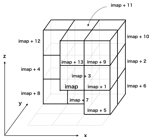
図 3.2 隣接セルのマッピング：中央のセル \text{imap} が参照する隣接セルのインデックスを \text{imap}+1 から \text{imap}+13 まで割り振る．作用反作用の法則から参照セルは対角方向のみを割り当てれば良い．
