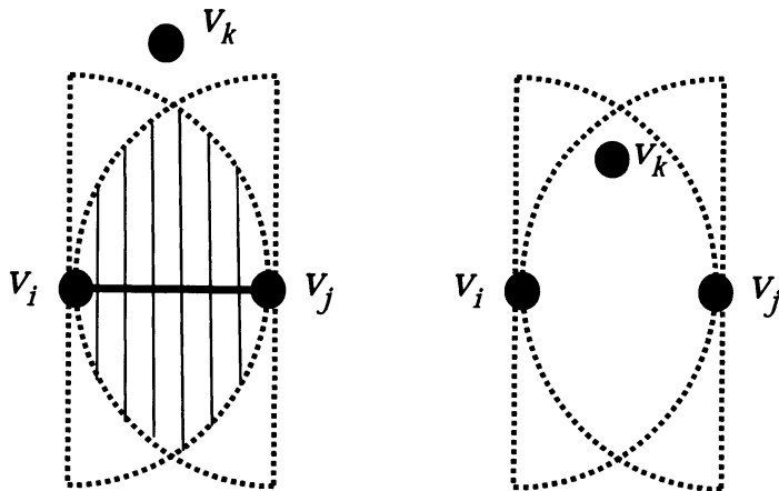
図 2: 相対近傍グラフにおける辺の判定
