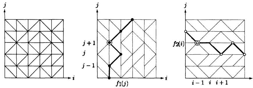
図 4: 一般の単体分割の場合の最適応答
