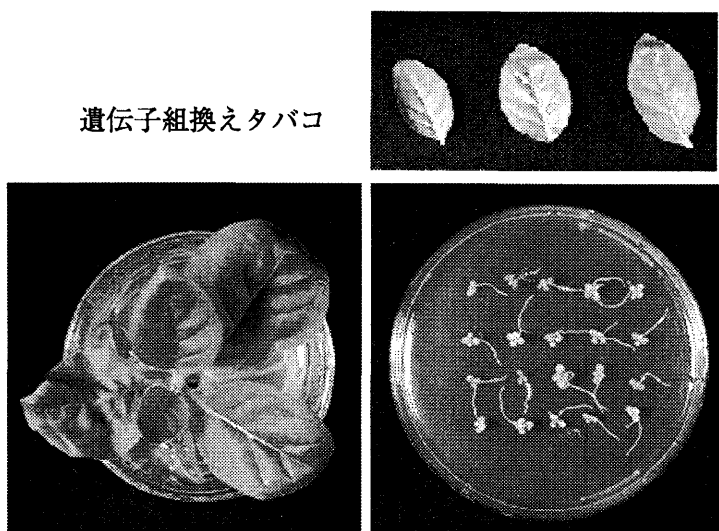
図 4. ABC トランスポータ遺伝子の導入されたタバコ
