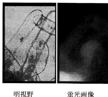
図 5. ダウノルビシンは hMRP1 発現タバコの液胞に貯まる
