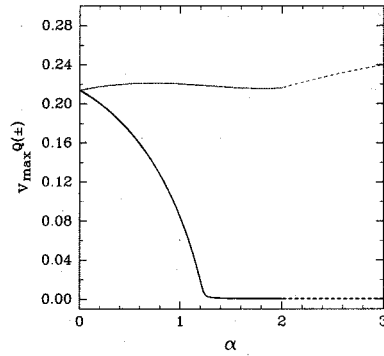
図2 局所性関数 L_{\alpha}^{Q(\pm)}(v) が最大となる波数比 v_{\max}^{Q(\pm)} の \alpha 依存性. 太線は v_{\max}^{Q(+)} を, 細線は v_{\max}^{Q(-)} を表す. 図1と同様に \alpha > 2 ではエンストロフィースペクトルのスケーリング則の導出に失敗しているので, 参考のために点線で記している.
