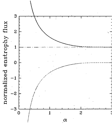
図1 エンストロフィー散逸率で規格化したエンストロフィー慣性領域のエンストロフィーフラックスの \alpha 依存性. 太線は \Pi_{\alpha}^{Q(+)}(k)/\eta_{\alpha} , 細線は -\Pi_{\alpha}^{Q(-)}(k)/\eta_{\alpha} , 一点破線は正味のエンストロフィーフラックスである. \alpha > 2 ではエンストロフィースペクトルのスケーリング則の導出に失敗しているので, 参考のために点線で記している.
