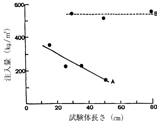
図11 圧縮処理したカラマツ心材への注入量 42)
