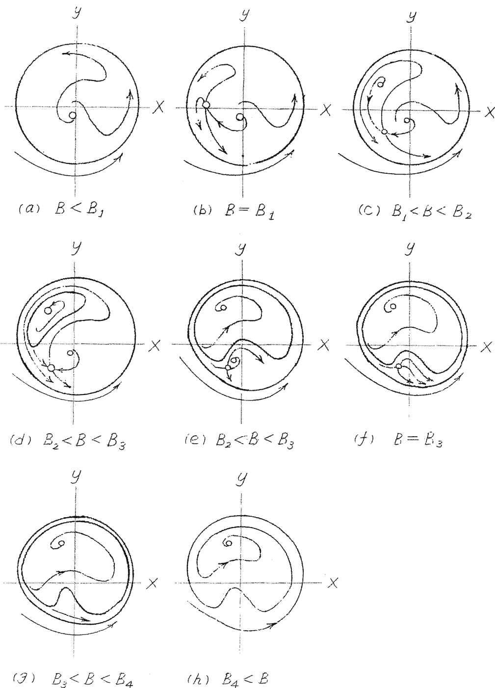
第5図 外力周波数 \nu を一定とし、振巾 B をかえた場合の同期振動と概同期振動相互間の関係を示す積分曲線の模様
