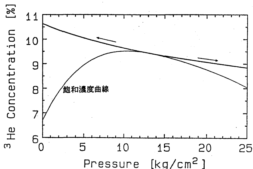
図3 ^3\text{He} 希薄相 (d 相) での ^3\text{He} 濃度の圧力依存性 ( x_d - P 図)
