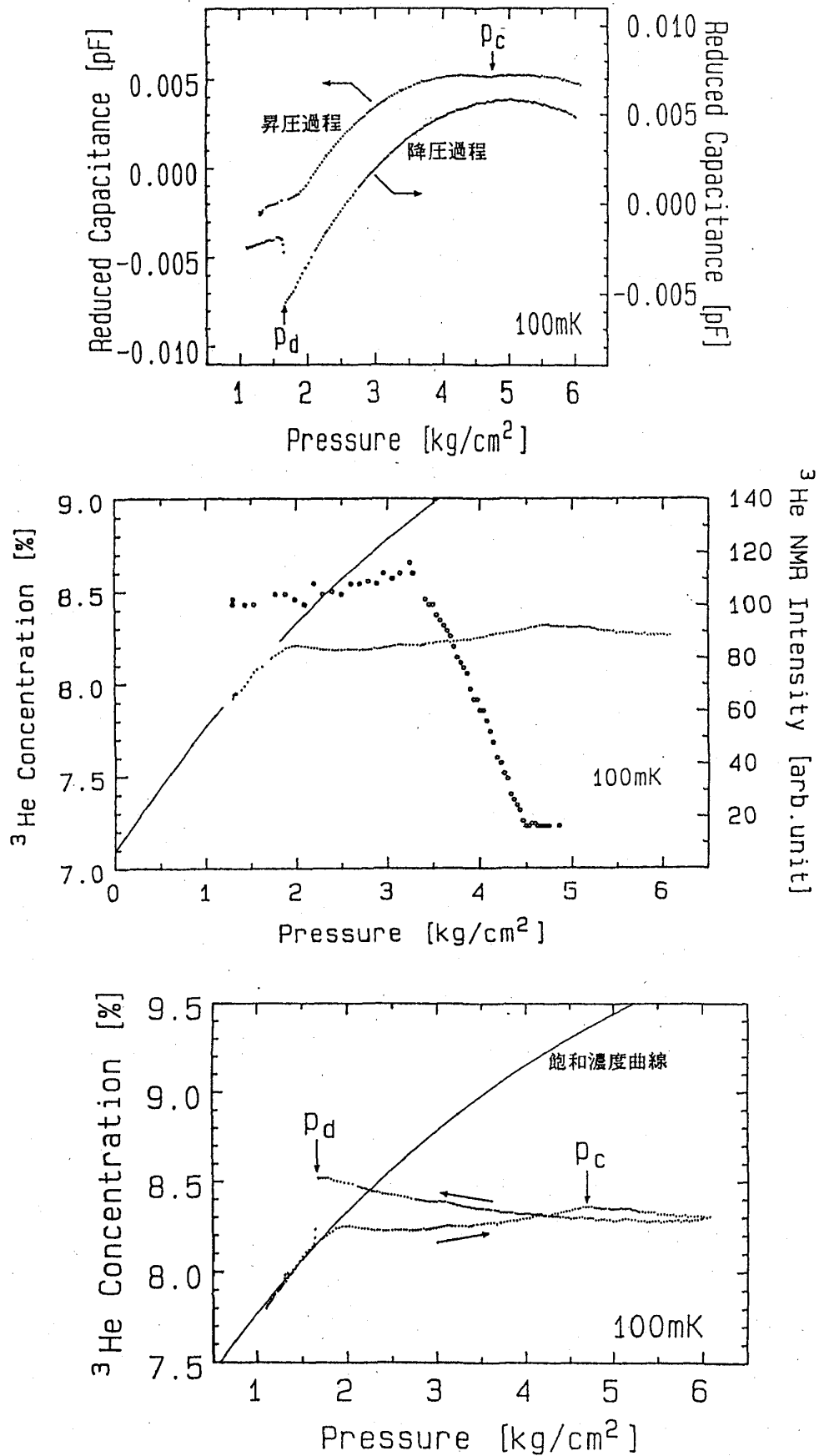
図8 100mK での測定データ (a), (b), (c)の説明は図7の場合と同じ
