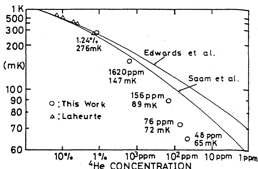
図10 ^3\text{He} 濃厚相 (c 相) 中の ^4\text{He} 濃度の温度依存性 [11]
