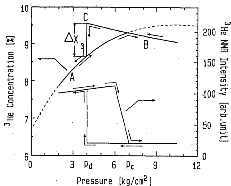
図5 図4に対応する x_3 - P 図と ^3\text{He} NMR 強度の変化
