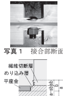
図9 接合部断面
