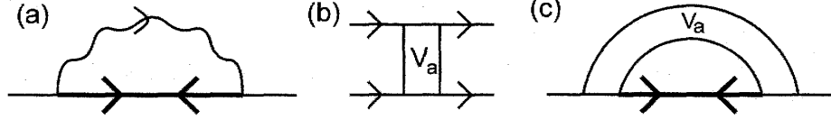
図 8 (a) 異常自己エネルギー \Delta(k) に対する電子格子相互作用の 1 ループ項。波線はフォノンのグリーン関数を表している。(b) 粒子・粒子チャンネルの既約 4 点バーテックス。(c) 既約 4 点バーテックスを用いた異常自己エネルギーの表示。
