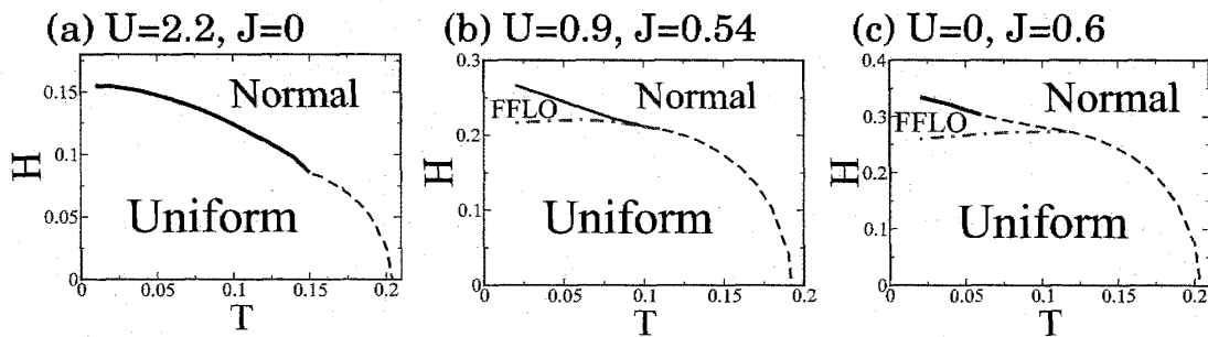
図 21 スピン相関によって高磁場の超伝導相図が変更を受けることを示す計算結果 [66]。(a) スピン相関が局所的な場合。(b) スピン相関がやや反強磁性的な場合。(c) スピン相関が反強磁性的な場合。点線は二次転移、実線は一次転移を表す。
