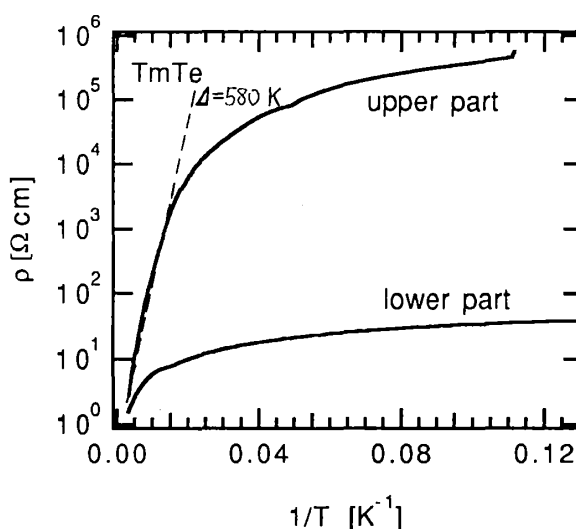
Fig.2.2 電気抵抗の \log \rho - 1/T プロット。Δは \rho \propto \exp(\Delta/T) の式による。
