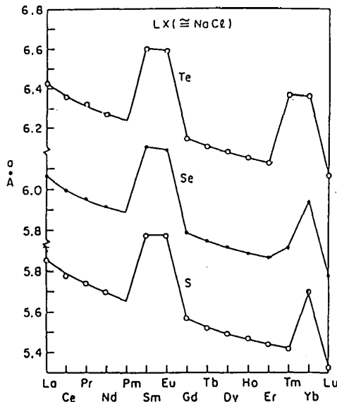
Fig.1.1 稀土類モノカルコゲナイドの格子定数 ([1]より転載)。
