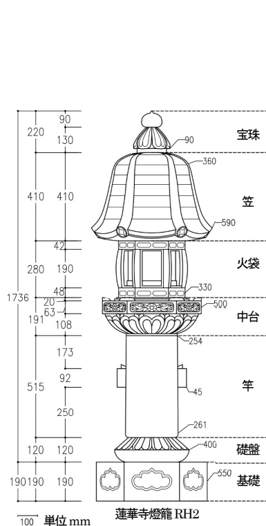
図一 蓮華寺燈籠の見取り図
